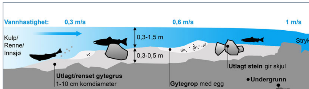
Figur 15. Restaurert gyteplass for laks sett i lengdeprofil med typiske egenskaper. Grusen er lagt ut på et typisk «brekk» i overgangen fra kulp, renne eller innsjø til nedenforliggende strykparti. En slik plassering gir gunstige hydrauliske forhold for gyting.
