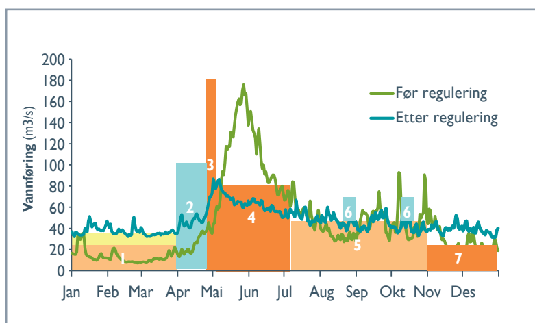
Figur 12. Eksempel på byggeklossmetoden med vannføringskurve før og etter regulering og viktige vannføringsbokser. Varighet (x-aksen) og vannføring (y-aksen) gir vannslippets størrelse (areal av boksene) som samlet summeres til strekningens vannbank. 1=eggoverlevelse og vinterhabitat, 2=smoltutvandring, 3=spyleflommer, 4=ungfiskvekst, 5=ungfiskhabitat, 6=lokkeflommer for fiske/gytevandring, 7=gyting. Fargene angir prioritering (fra orange som er høyt prioritert til blått som er lavt prioritert) ut fra identifiserte hydrologiske flaskehalsar og styrken av disse.
