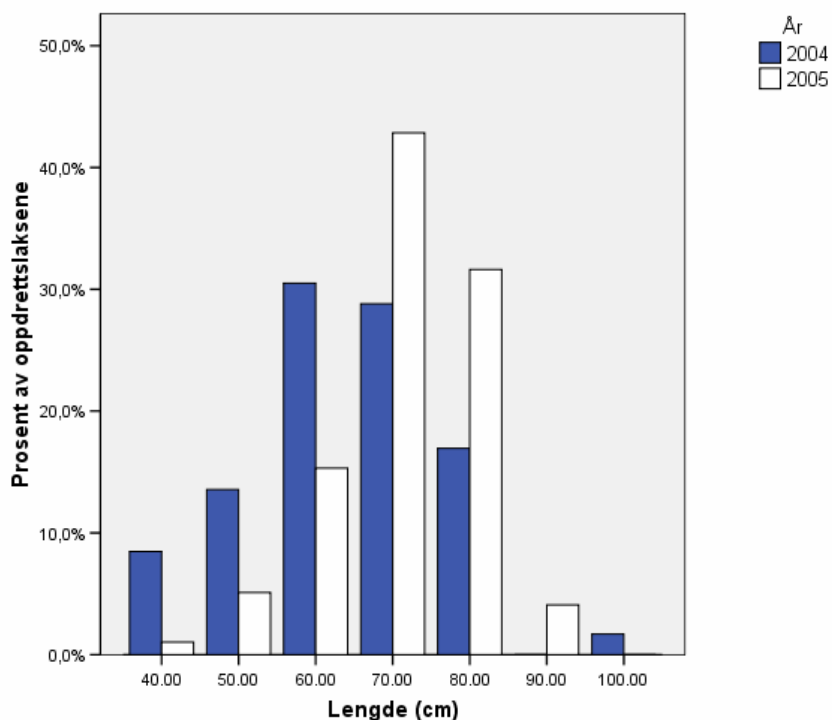
Figur 3. Lengdefordeling (10 cm intervaller) av rømt oppdrettslaks fanget i Salvassdraget i 2004 (n = 59) og 2005 (n = 98).
