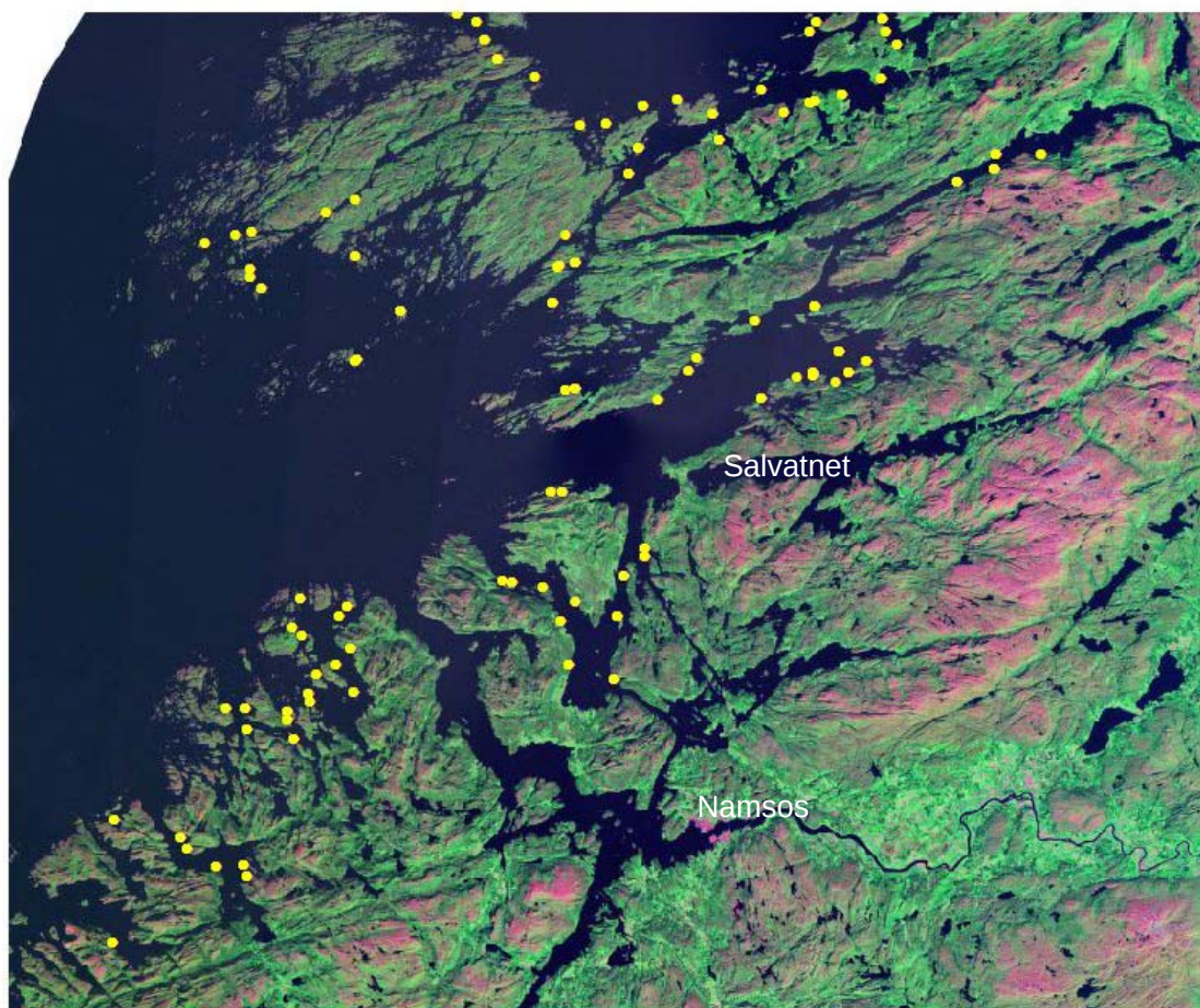
Figur 1. Lokaliteter for mattiskanlegg for laksefisk i Namdalsområdet plottet på satellittfoto over området. Gule prikker viser godkjente lokaliteter per 1. januar 2004 (både lokaliteter som er i bruk og lokaliteter som ikke er i bruk). Kilde: Fiskeridirektoratet.
