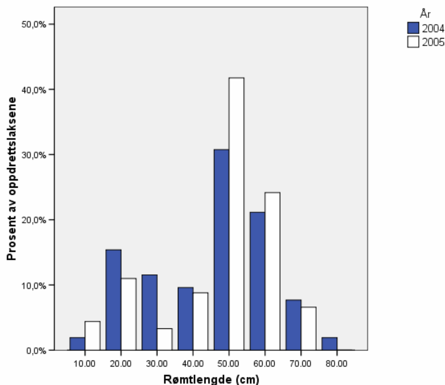
Figur 4. Tilbakeberegnet kroppslengde ved rømming (10 cm intervaller) for rømt oppdrettslaks fanget i Salvassdraget i 2004 (n = 52 som hadde skjell med så liten erosjon at de kunne brukes til tilbakeberegning) og 2005 (n = 91).
