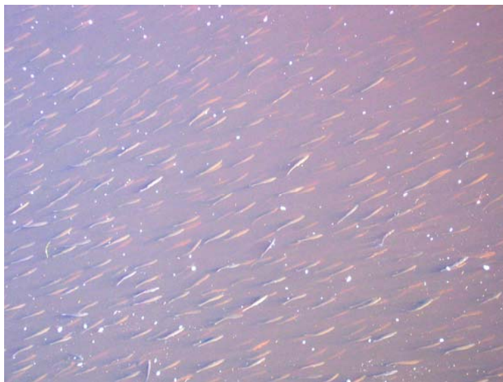
Bilde 1: Mort på gytevandring inn i Åkersvika. Bildet er tatt fra Stangebrua den 19. mai 2005. I følge Huitfeldt-Kaas (1918) gikk morten opp i Svartelva for å gyte omkring 25. mai eller sitat: "Naar heggeblomsten begynner å springe ut gaar sørennen (mort) op i Svartelven, det er et gammelt merke som aldri slår feil" (foto: J. Museth)
