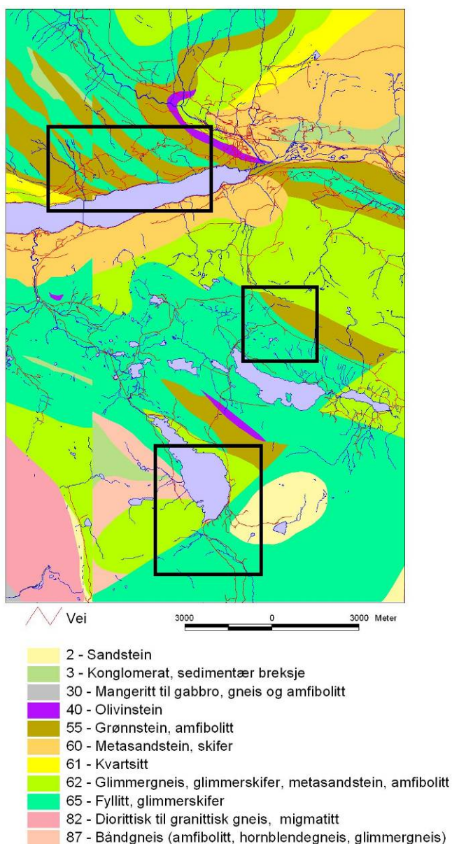
Figur 4. Berggrunnsgeologien rundt de tre undersøkelsesområdene i Vågå (Fra Norges Geologiske Undersøkelse: www.ngu.no )
