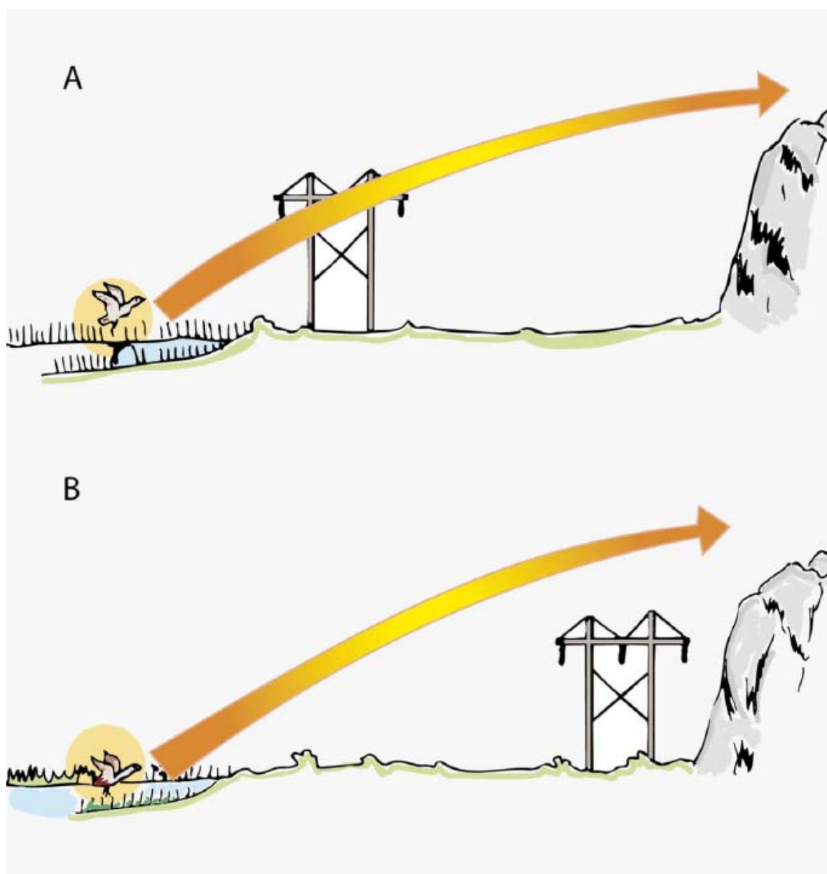
Figur 14. Topografiske strukturer som tvinger fugler til å fly over kraftledningen reduserer faren for at fugler skal kollidere med linene. A viser uheldig lokalisering sammenlignet med B. Omarbeidet etter Thompson (1978).
