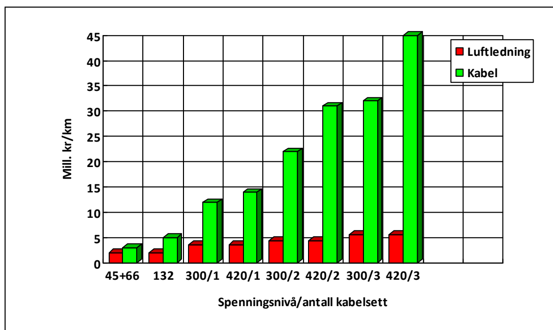
Figur 22. Totale kapitaliserte kostnader ved et valgt overføringsnivå for ulike spenningsnivåer og ulike antall kabelsett (300 og 420 kV) (etter Trohjel & Vognild 1993).
