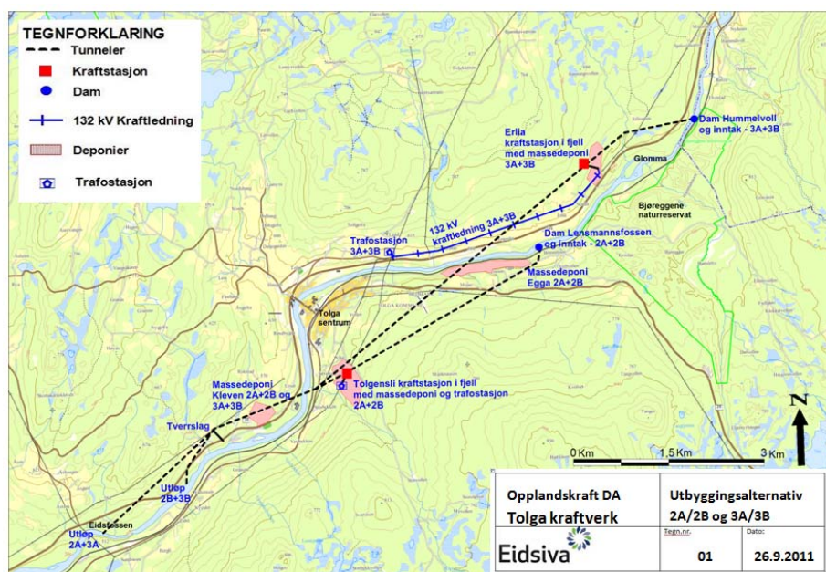
Figur 1.1 Oversiktskart med de endelige alternativene for utbygging av Tolga kraftverk (kilde: Opplandskraft)
