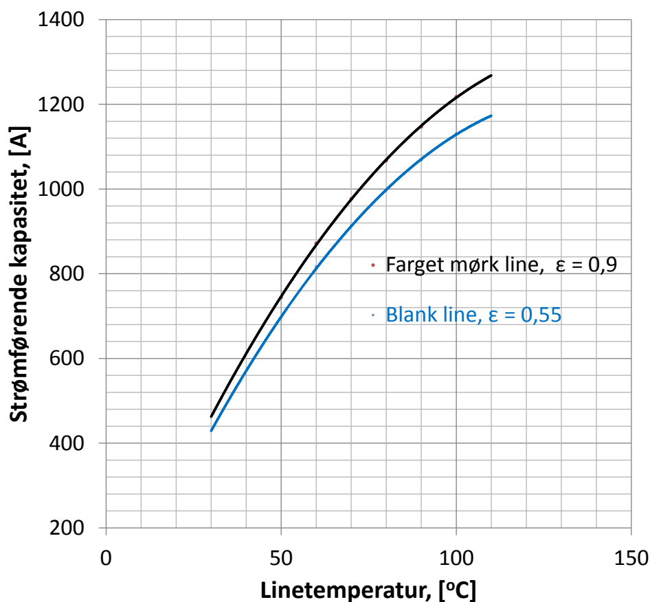
Figur 9. Strømførende kapasitet til blanke stålaluminiumliner ( \varepsilon = 0,55 ) og fargede liner ( \varepsilon = 0,90 ) av typen FeAl 240-26/7. Vindhastighet = 0,6 m/s, omgivelsestemperatur 20°C, solinnstrålingsintensitet 900 W/m 2 .
