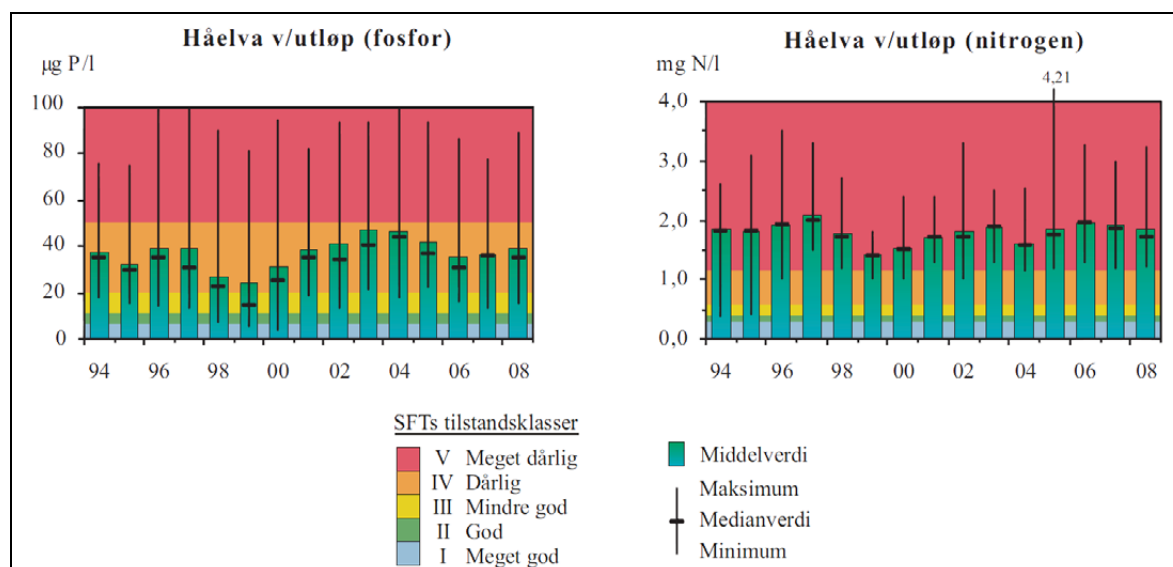
Figur 7. Vannkvaliteten ved utløpet av Håelva angitt ved total fosfor og total nitrogen i perioden 1994-2008. Fra Molversmyr (2009).
