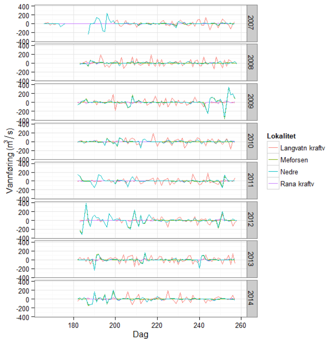
Figur 6. Endring i vannføring (fra dagen før) ved ulike lokaliteter i Ranaelva gjennom fiske-sesongen. Døgngjennomsnittene vist i figur 5 ligger til grunn for denne figuren.
